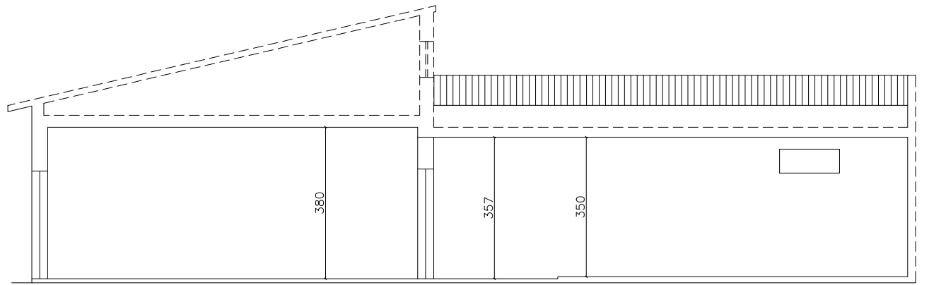
SEZIONE X-X
